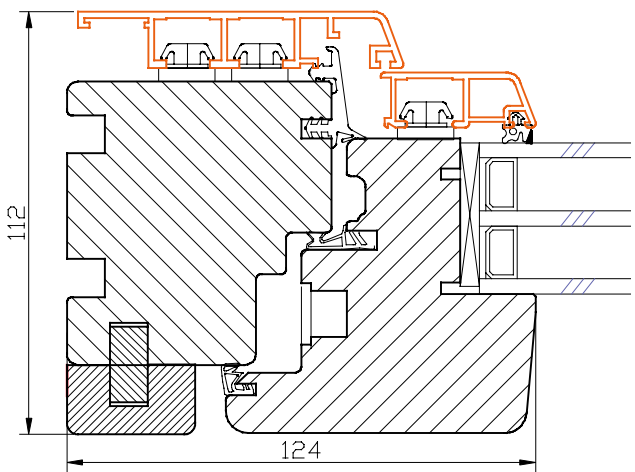
B-B (1:2)
