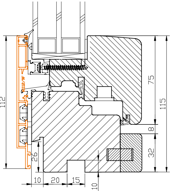
B-B (1:2)
