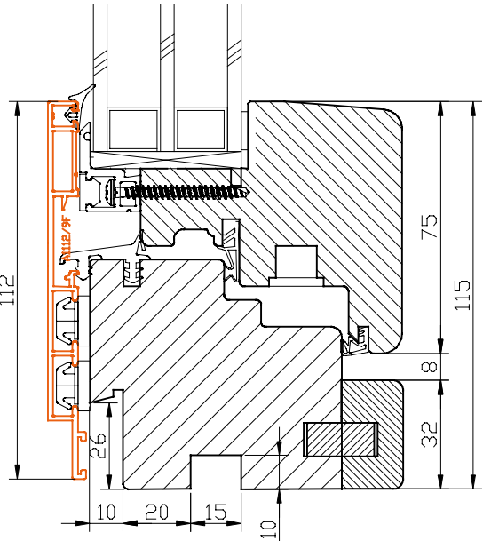
B-B (1:2)
