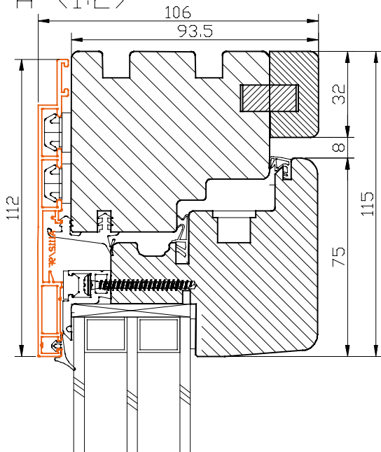
A-A (1:2)
