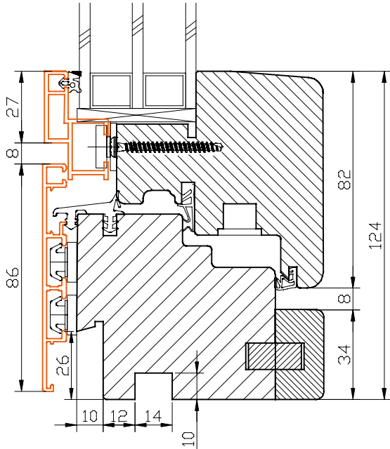
B-B (1:2)
